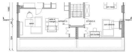
Plan du deuxième étage - 1/100
